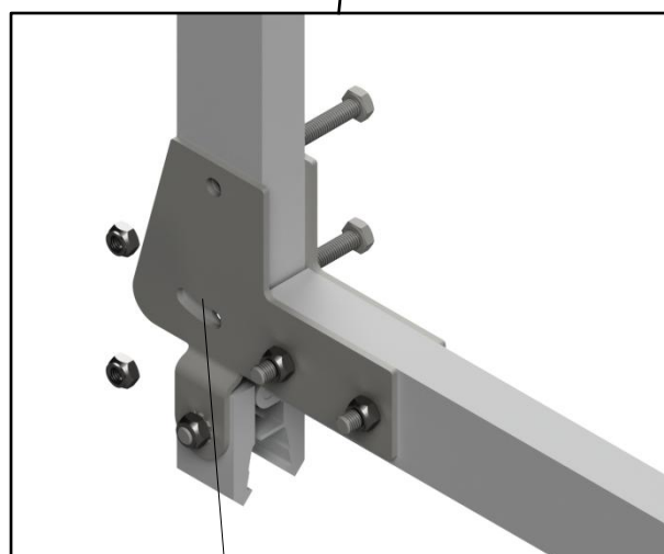
Dettaglio A
