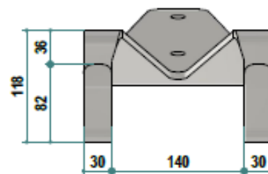
VISTA FRONTALE
