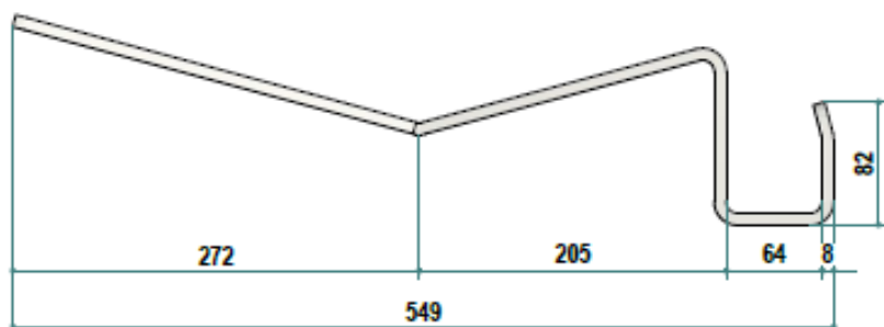
VISTA LATERALE
