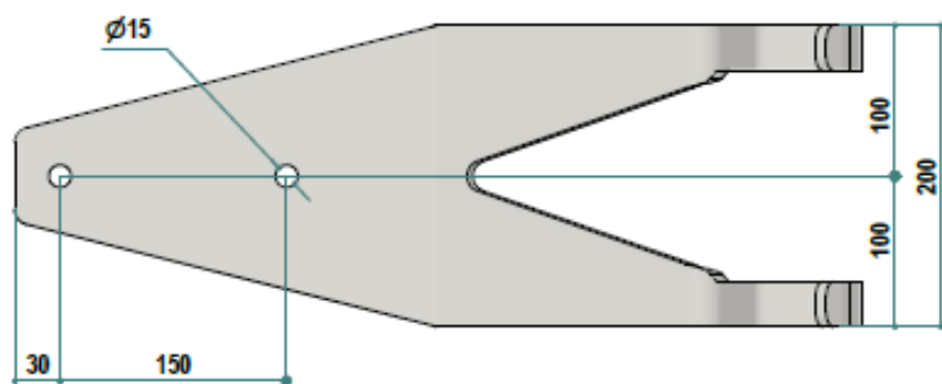
VISTA SUPERIORE
