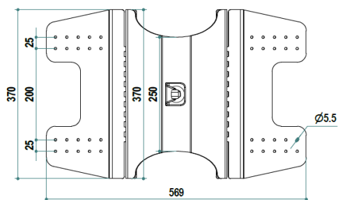
VISTA SUPERIORE
