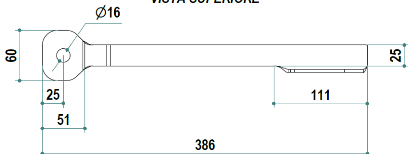
VISTA SUPERIORE
