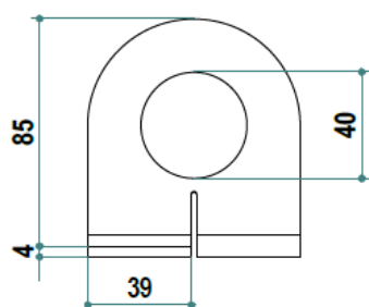
VISTA FRONTALE
