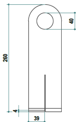
VISTA FRONTALE
