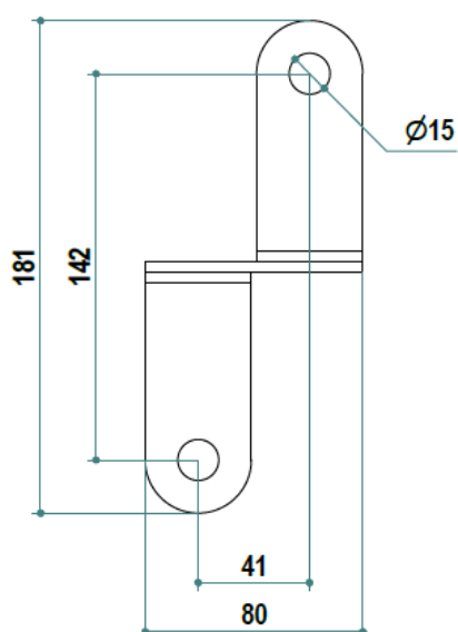
VISTA SUPERIORE
